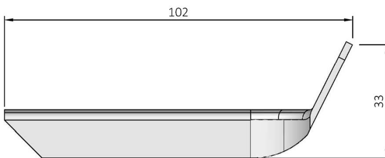
Unterteil "XU900"
